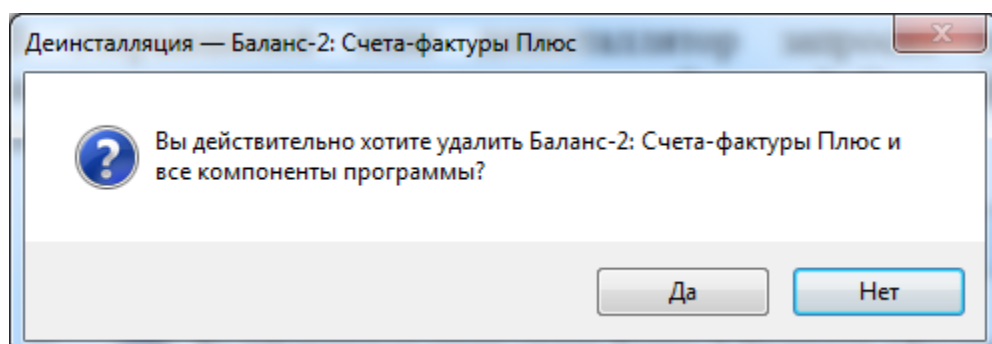
Рис.10. Окно деинсталляции
